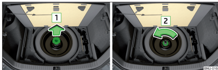
Obr. 317 Vyjmutí kola
