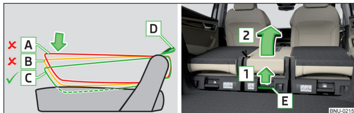
Obr. 90 Vyklopení prostředního sedadla
