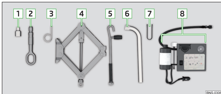
Obr. 316 Palubní nářadí
