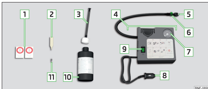
Obr. 324 Popis sady na opravu pneumatik
