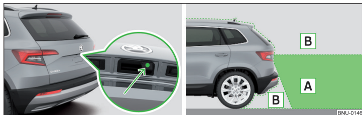
Obr. 269 Umístění kamery / Snímaná oblast za vozidlem
