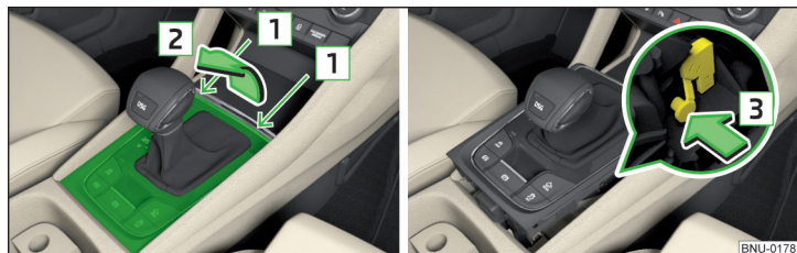
Obr. 335 Vyjmutí krytu / Odblokování volicí páky
