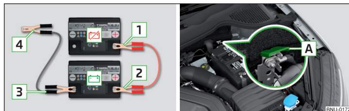
Obr. 325 Pomoc při startování: ☒ - vybitý akumulátor, ☐ - pomocný akumulátor / Kostiční bod motoru u systému START-STOP
