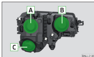
Obr. 345 Levý přední světlomet
