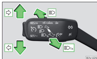
Obr. 62 Ovládací páčka: ovládání směrových a dálkových světel
