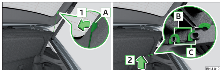
Obr. 143 Vyjmutí krytu zavazadlového prostoru
