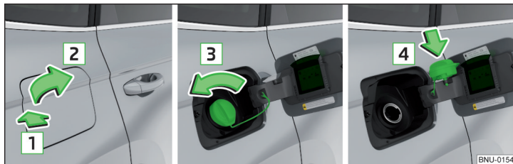
Obr. 301 Odklopení krytu hrdla palivové nádrže / Vyšroubování uzávěru / Nasazení uzávěru na kryt
