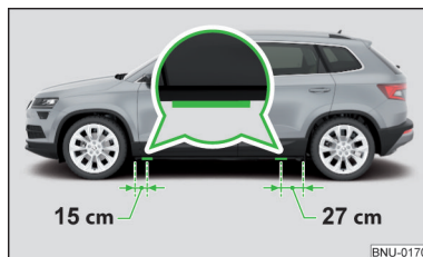
Obr. 322 Výztuhy pro nasazení zvedáku vozidla
