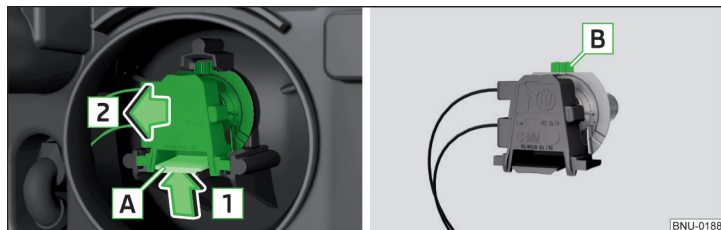
Obr. 346 Výměna žárovky potkávacího a dálkového světla
