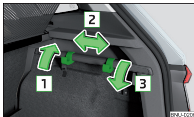
Obr. 139 Posun háčku po upevňovací tyči
