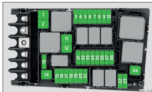
Obr. 344 Pojistky
