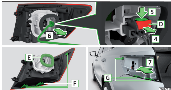
Obr. 352 Odpojení konektoru / Montáž svítliny
