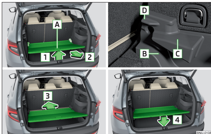
Obr. 154 Nastavení mezipodlahy
