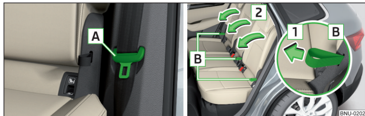
Obr. 88 Bezpečnostní poloha pásu / Sklopení zádové opěry
