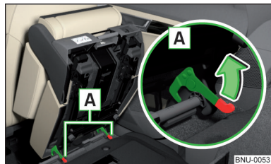
Obr. 93 Zajištění sedadla
