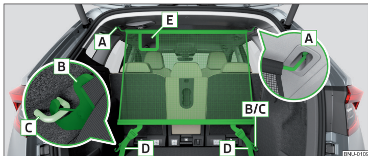
Obr. 147 Dělicí síť za zadními sedadly
