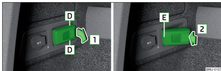
Obr. 153 Vyjmutí svítilny / Vložení svítilny
