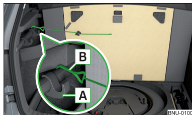
Obr. 142 Upevnění koberce
