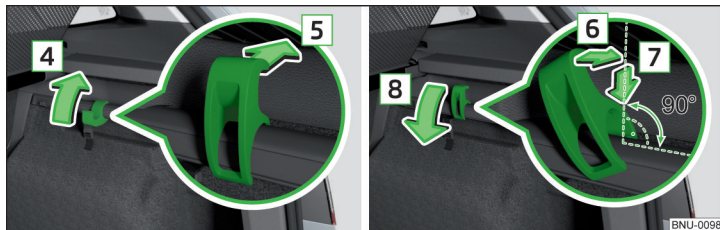
Obr. 140 Vyjmutí/vložení háčku
