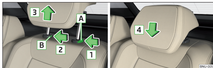
Obr. 97 Vyjmutí/vložení zadní hlavové opěrky
