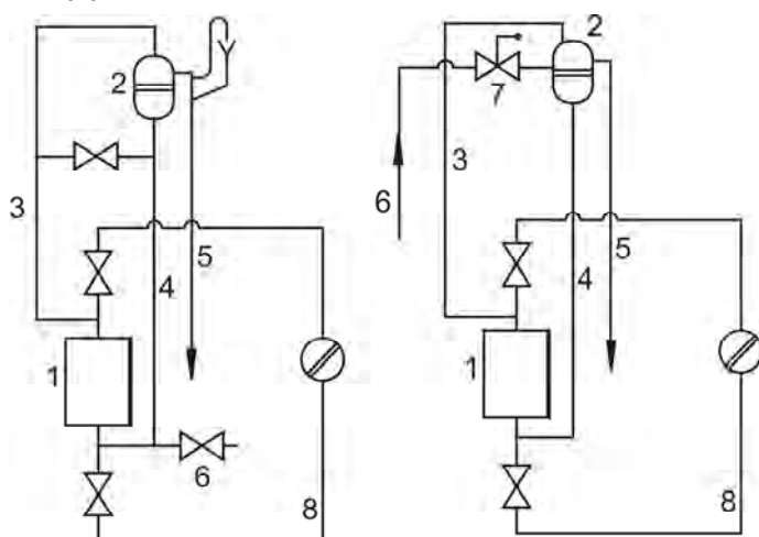
Obr. č. 10 Příklady zapojení otevřených expanzních nádob
