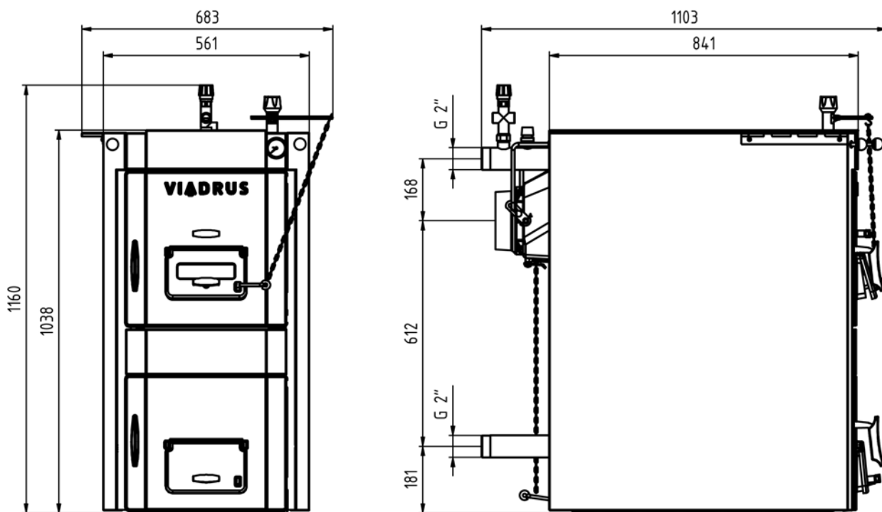
Obr. č. 2 Připojovací rozměry kotle HERCULES U 32
