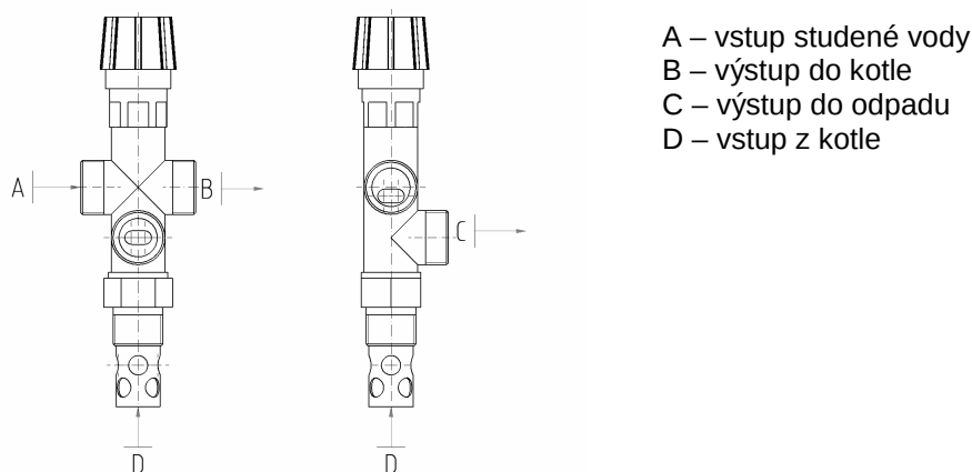
Obr. č. 8 Dvoucestný bezpečnostní ventil DVB 1 - 02
