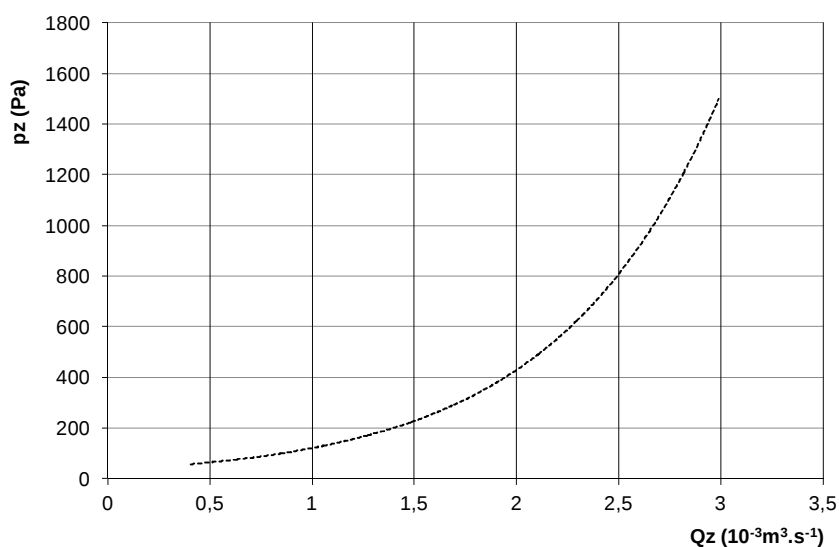
Obr. č. 1 Hydraulická ztráta kotlového tělesa
