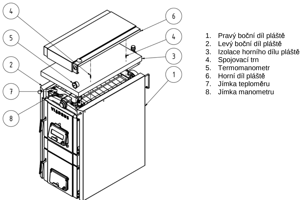
Obr. č. 25 Montáž horního dílu pláště
