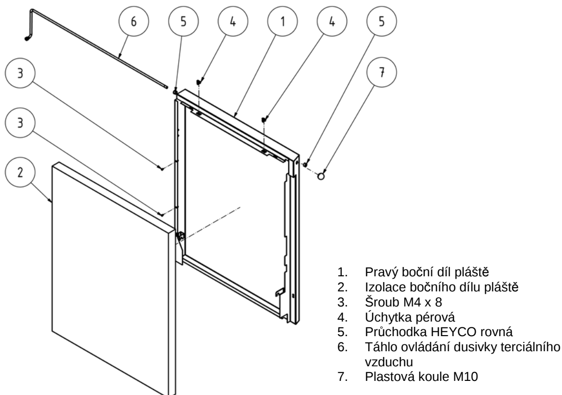
Obr. č. 23 Montáž táhla ovládání dusivky terciálního vzduchu
