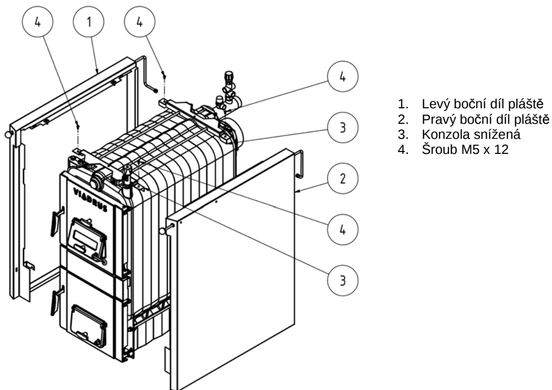
Obr. č. 24 Montáž bočních dílů pláště
