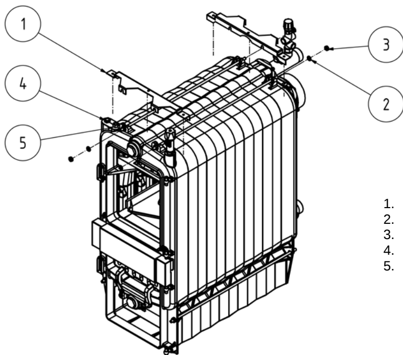
Obr. č. 21 Montáž konzol pláště
