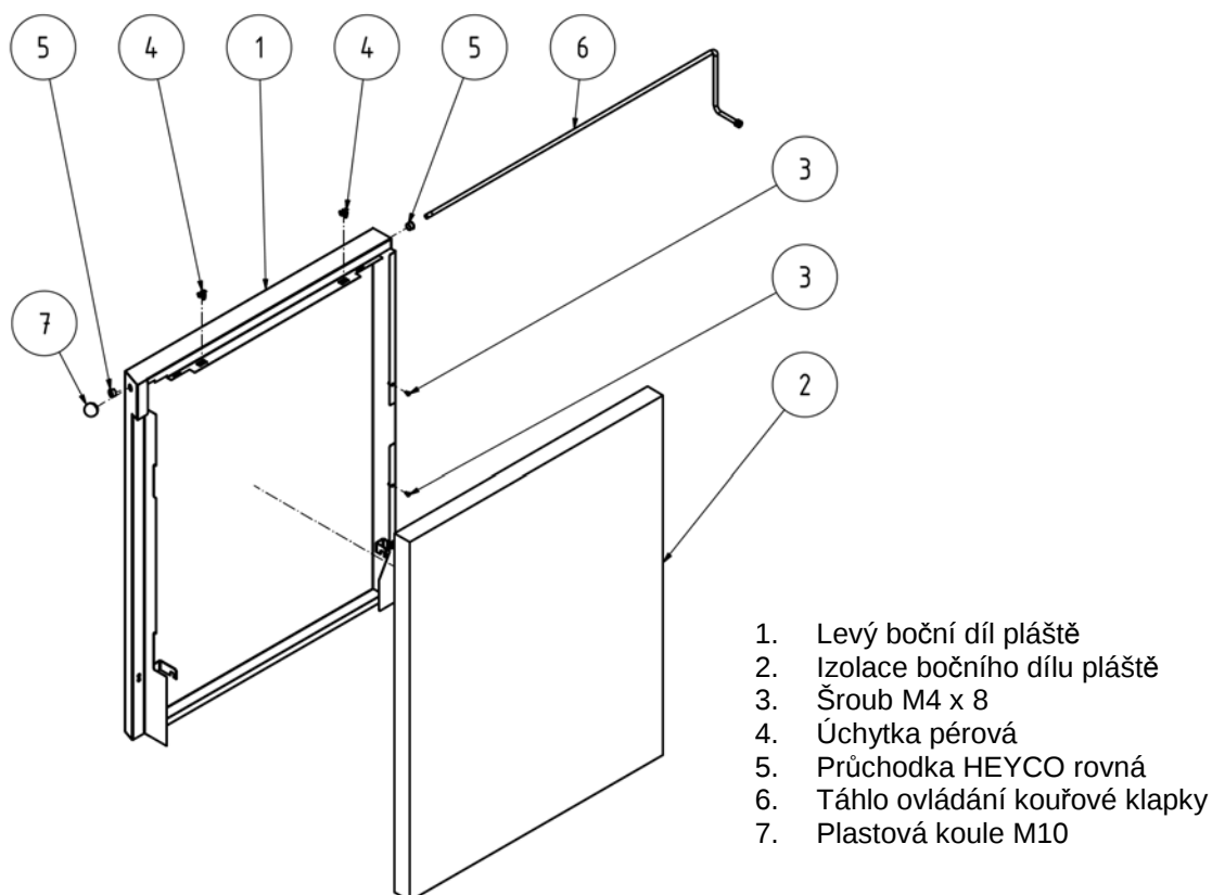
Obr. č. 22 Montáž táhla ovládání kouřové klapky
