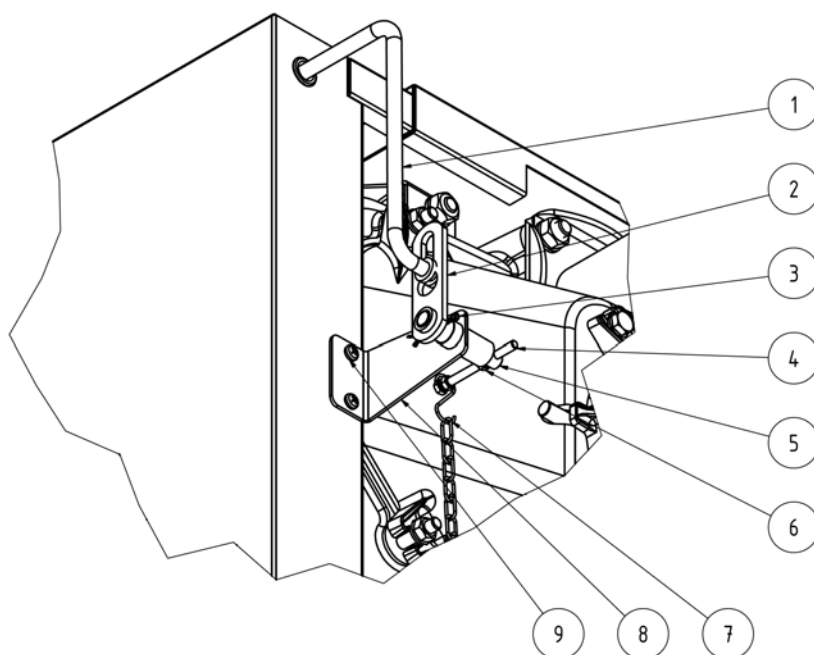
Obr. č. 29 Táhlo ovládání dusivky terciálního vzduchu
