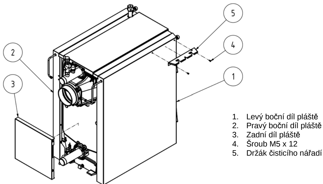
Obr. č. 26 Montáž zadního dílu pláště a držáku čistícího náradí
