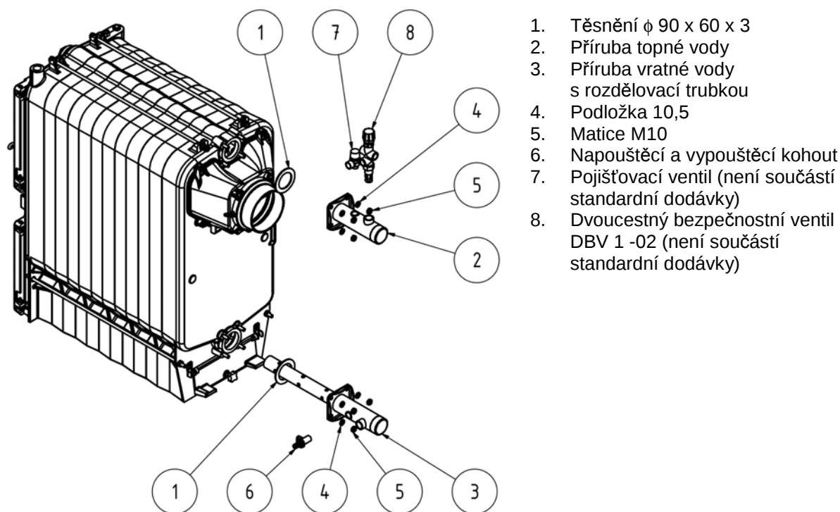
Obr. č. 14 Instalace kotlového tělesa
