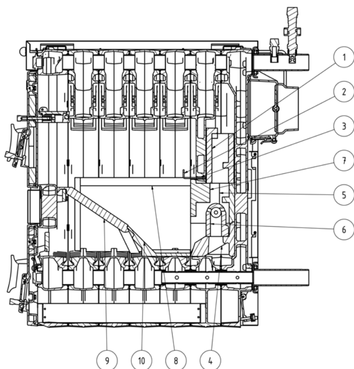
Obr. č. 18 Umístění keramických vložek do spalovací komory kotle HERCULES U 32 D - Dřevo
