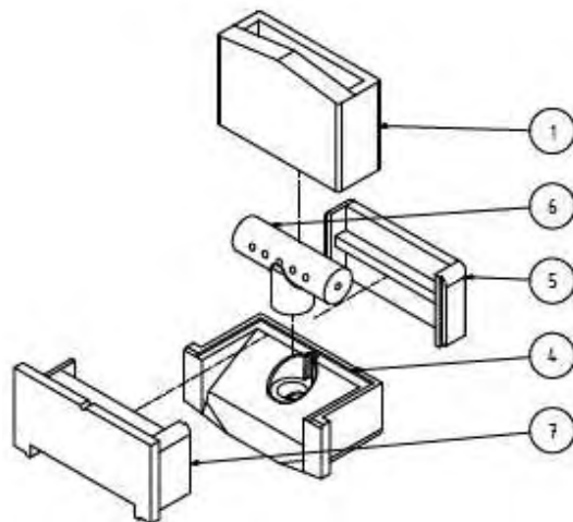
Obr. č. 19 Umístění keramických vložek do spalovací komory kotle HERCULES U 32 B a HERCULES U 32
