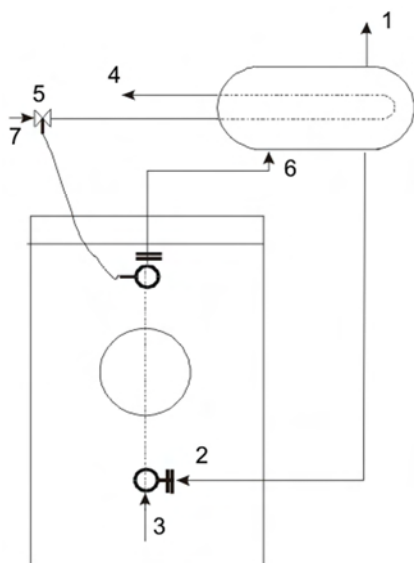
Obr. č. 7 Hydraulické schéma připojení dochlazovací smyčky
