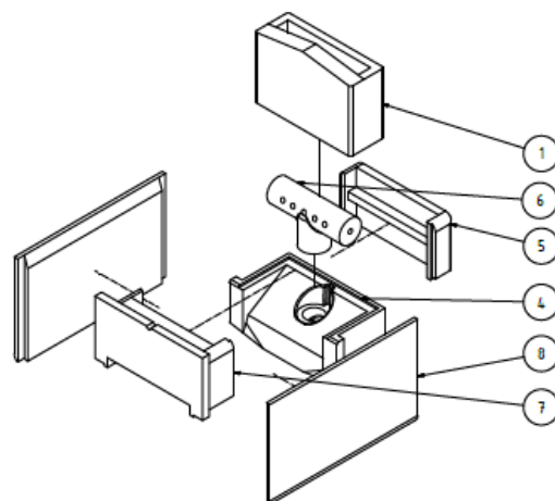
Obr. č. 18 Umístění keramických vložek do spalovací komory kotle HERCULES U 32 D - Dřevo
