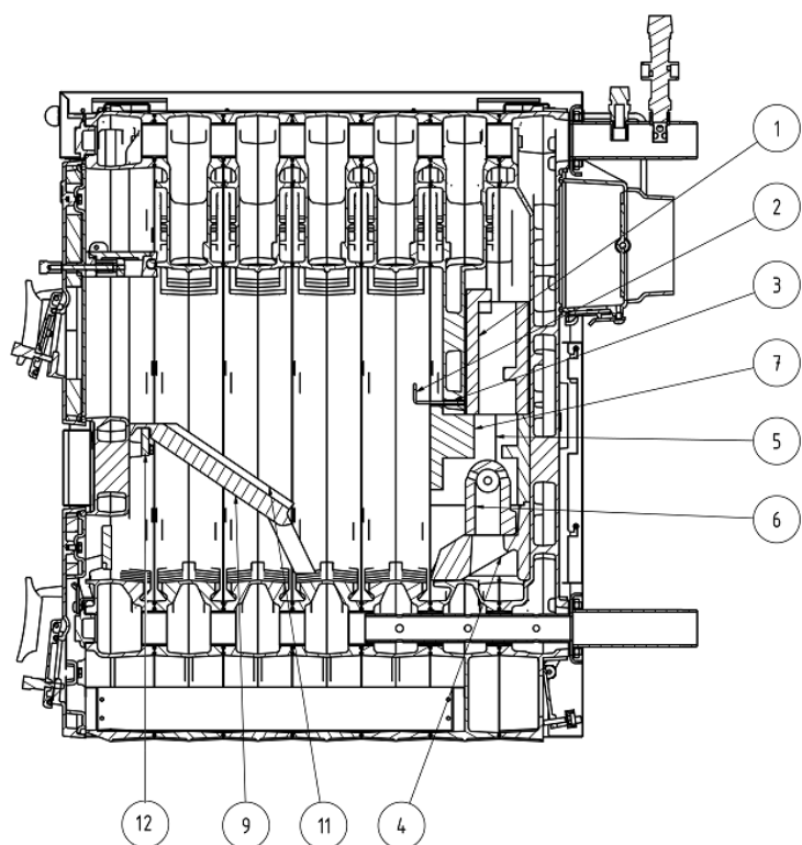
Obr. č. 19 Umístění keramických vložek do spalovací komory kotle HERCULES U 32 B a HERCULES U 32
