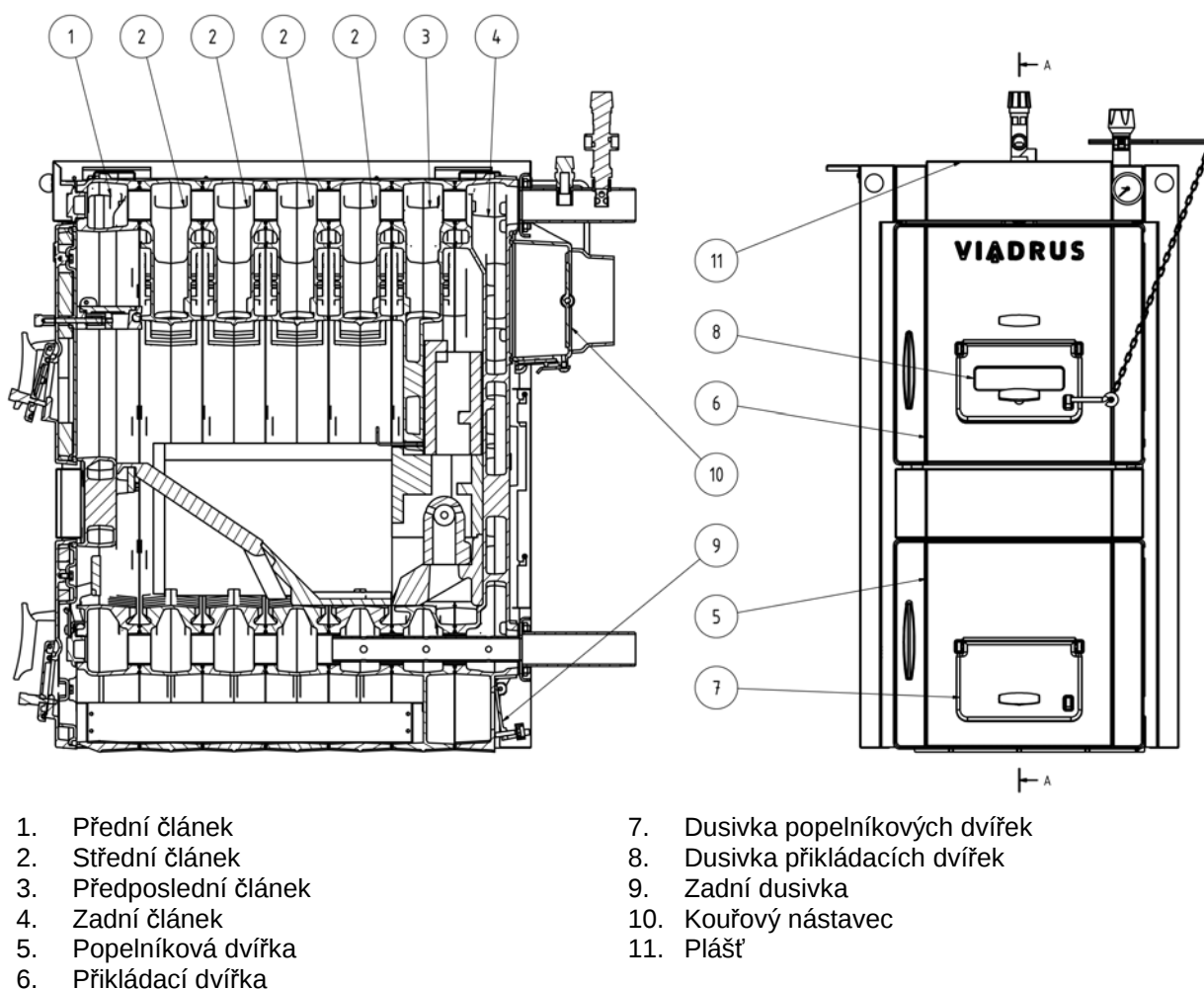
Obr. č. 3 Hlavní části kotle
