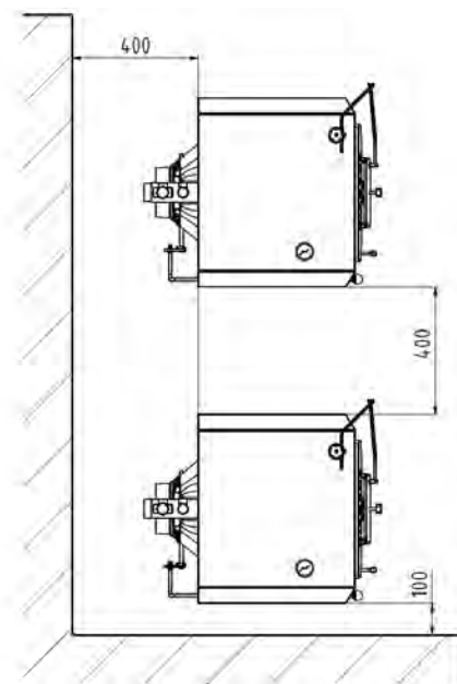
Obr. č. 13 Umístění kotlů v kotelně
