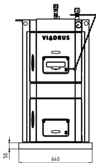
Obr. č. 11 Rozměry podezdívky
