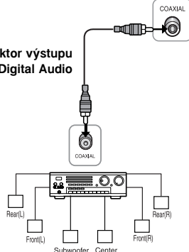
Ke vstupu Digital Audio Input přijímače A/V vybaveného funkcemi Dolby, MPEG2, DTS, Digital Decoder
