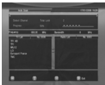
Obr. 4.2. Automatické hledání
