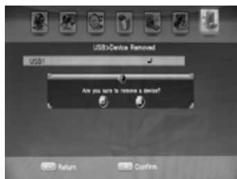
Obr. 5.7.3 Zařízení odpojeno
