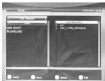
Obr. 5.6.3. Obraz zálohy
